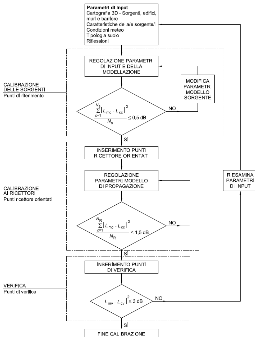
Figura 9 – Schema a blocchi esemplificativo di una possibile procedura di calibrazione (da [44]).
